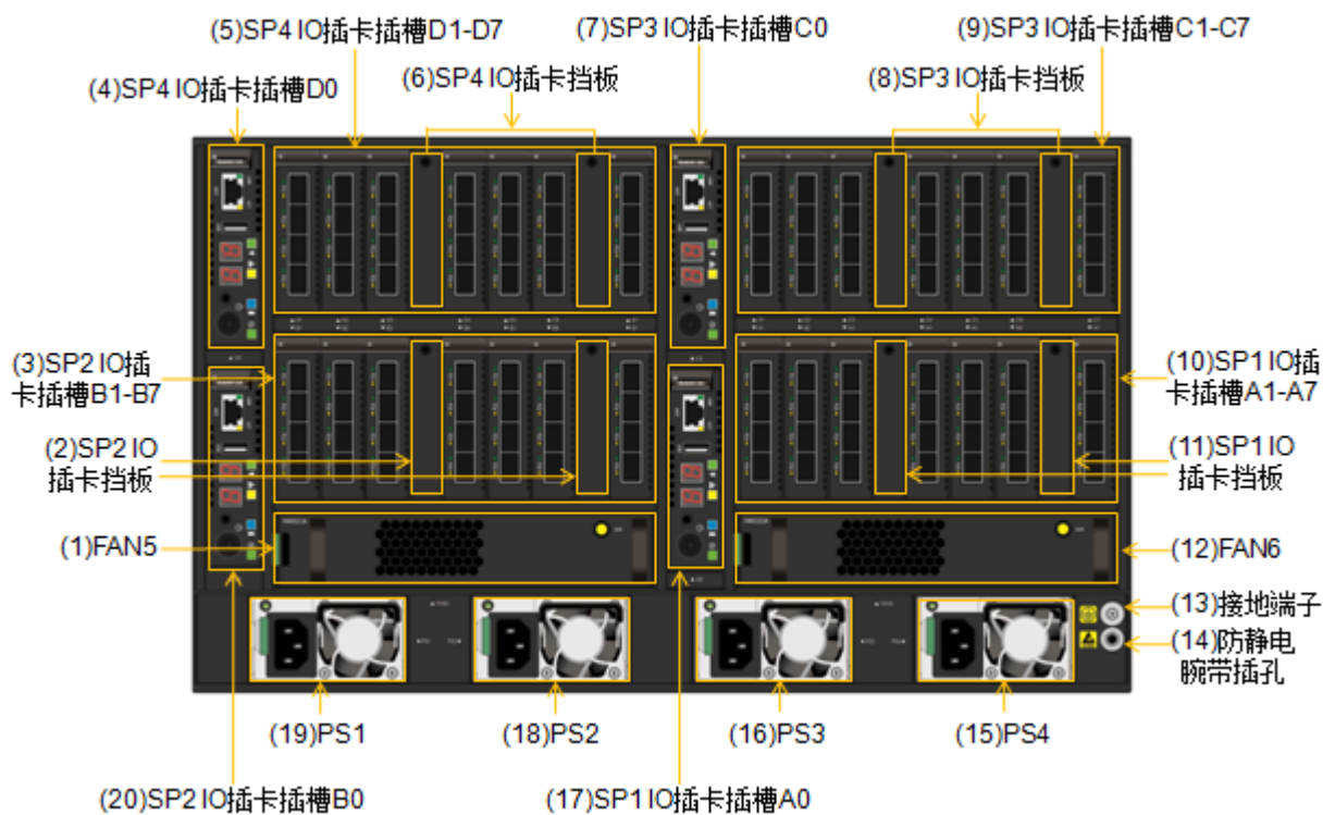
图3-3 SPU 后正视图
