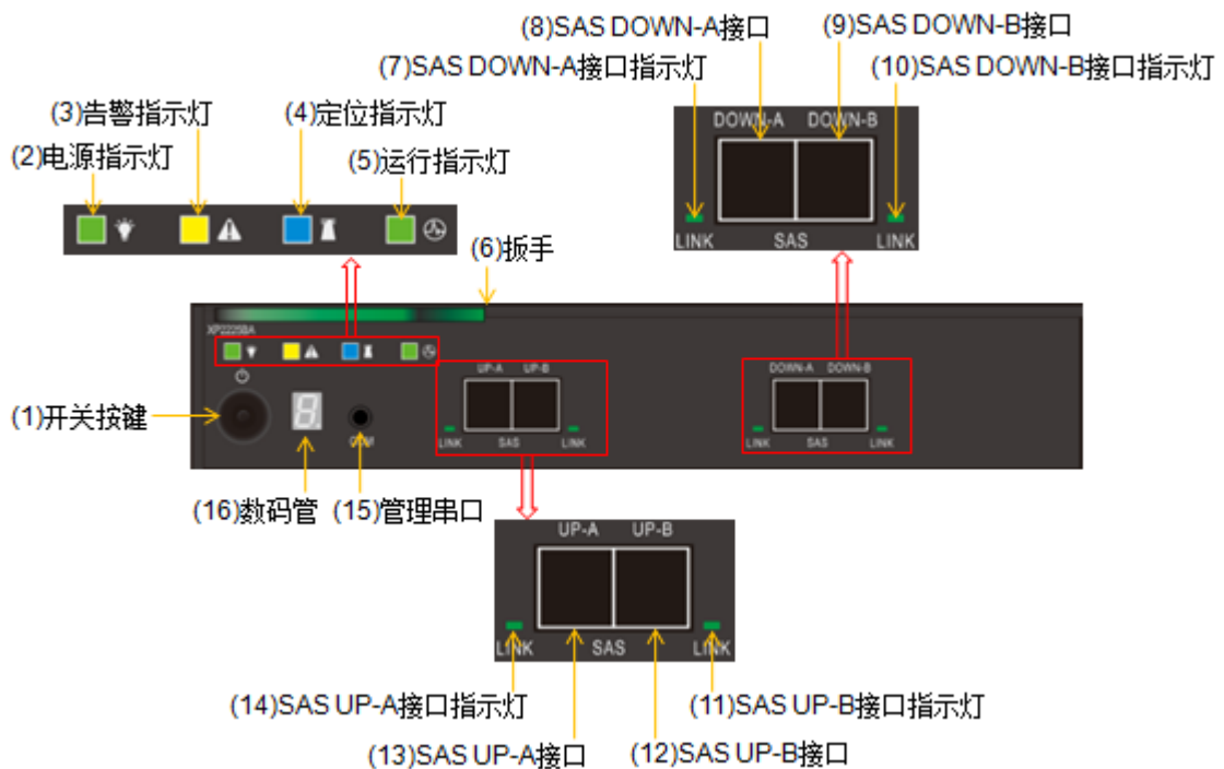
图3-13 SSU 的 XP 正视图
