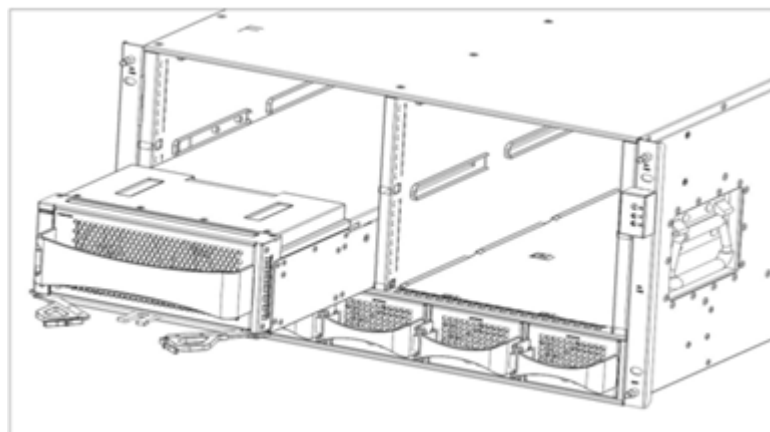
图4-14 安装 SP 示意图
