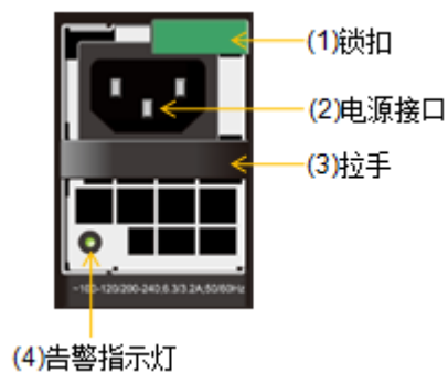
图3-21 DSU2625 电源模块正视图
