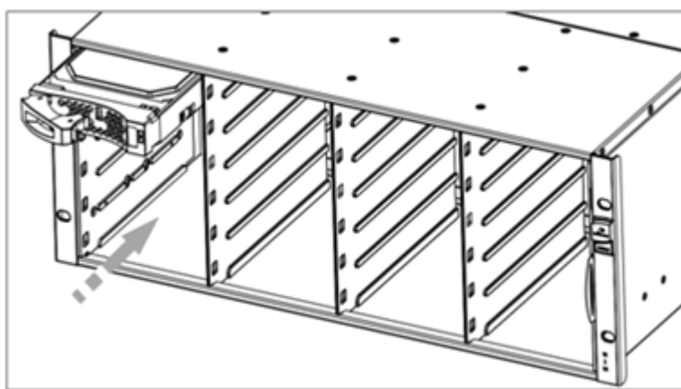
图6-22 安装 3.5 英寸磁盘模块示意图（二）
