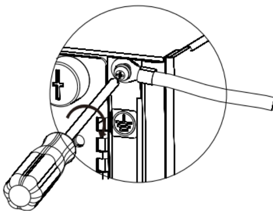
图4-30 安装接地线示意图
