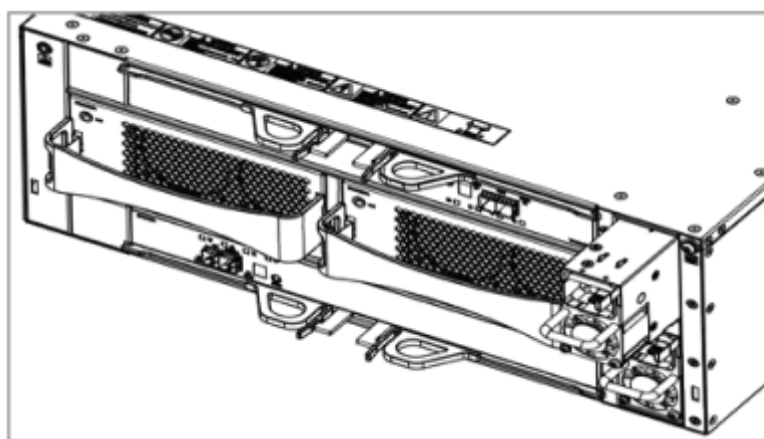
图6-14 安装/拆卸 DSU2624 电源模块示意图
