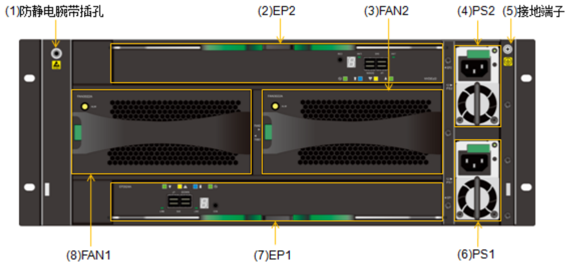
图3-23 DSU2624 后正视图
