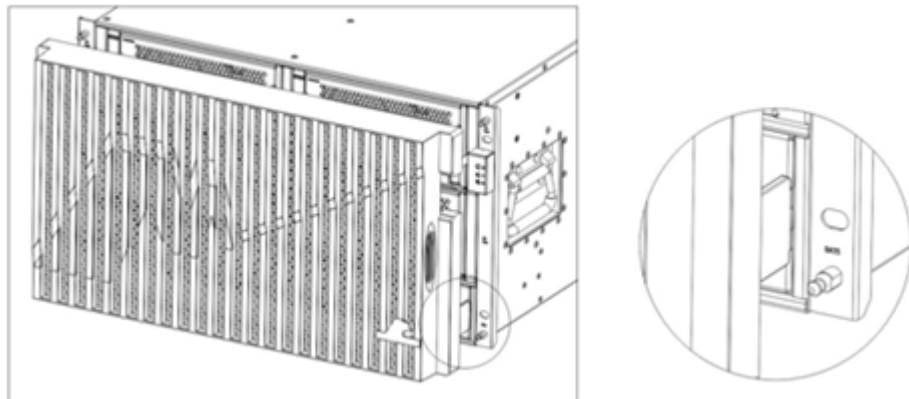
图6-1 安装/拆卸 SPU 面板示意图
