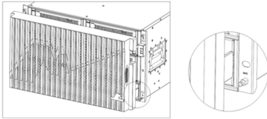
图4-16 安装 SPU 面板示意图
