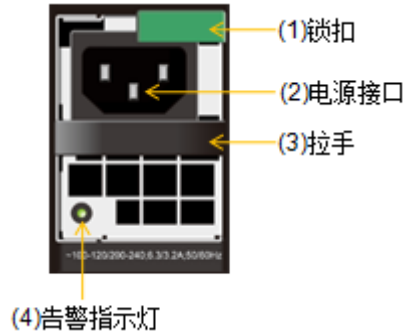
图3-16 SSU 电源模块正视图
