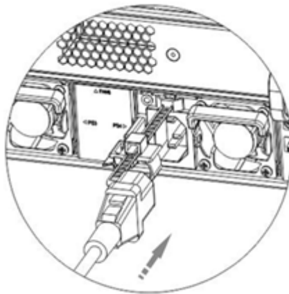
图4-32 安装电源线示意图（一）
