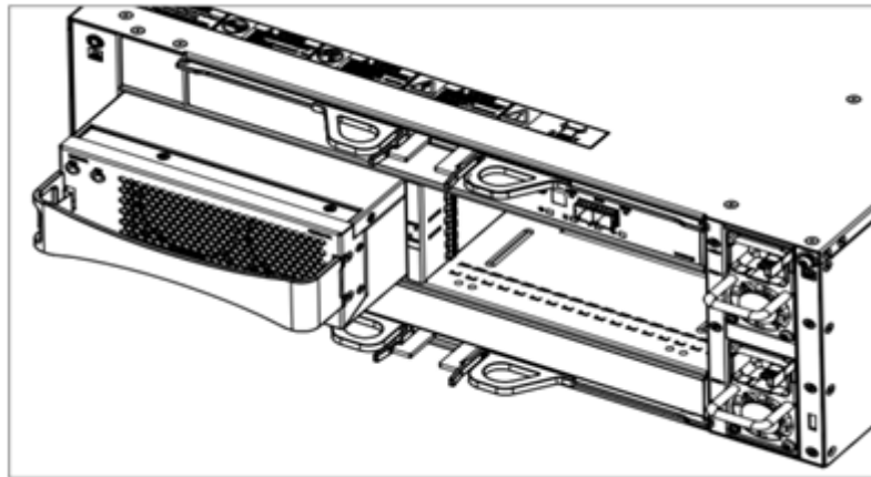
图6-13 安装/拆卸 DSU2624 风扇模块示意图
