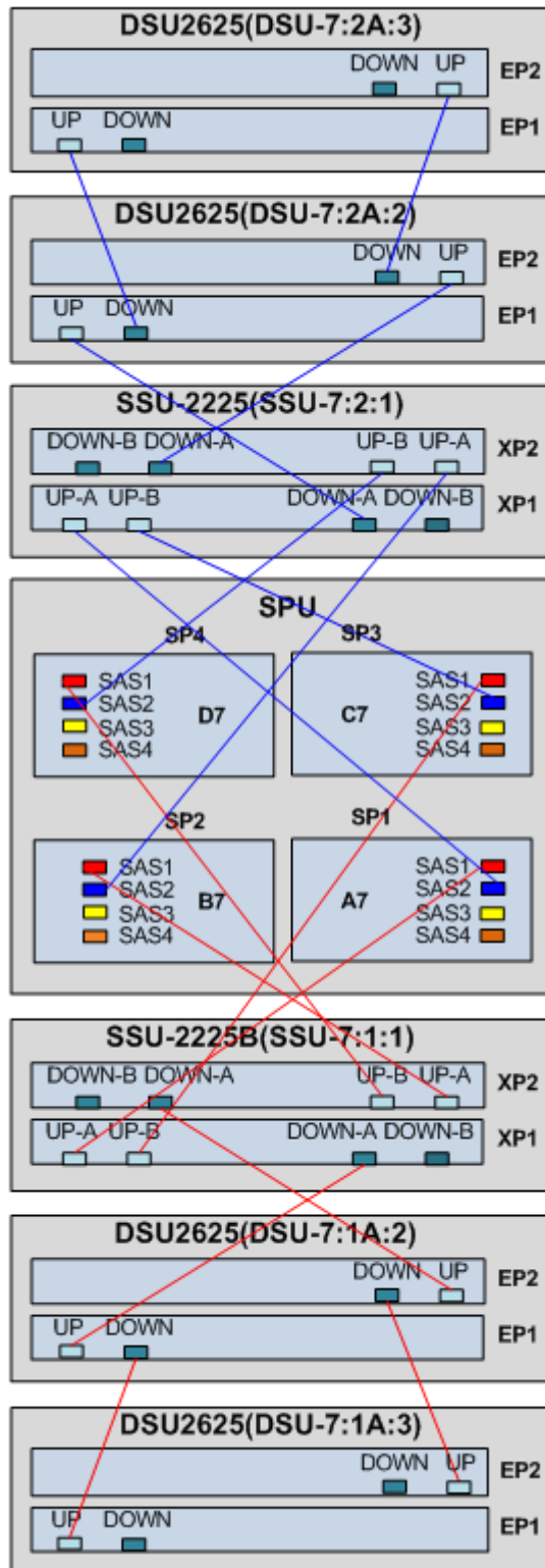
图4-40 SAS 线缆安装示意图
