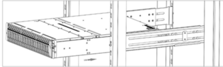
图4-18 安装 SSU2225B 示意图
