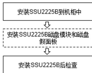
图4-17 SSU2225B 安装流程示意图
