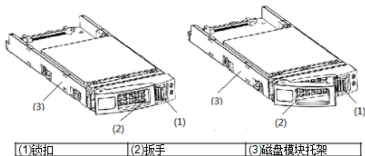
图6-15 2.5 英寸磁盘模块示意图
