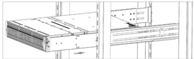
图4-20 安装 SSU2225 示意图
