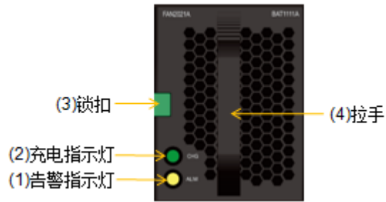
图3-14 SSU2225B 风扇模块+电池模块正视图
