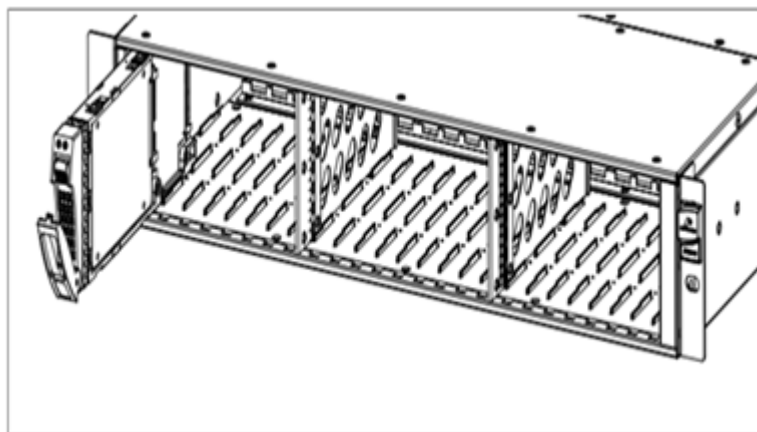
图6-18 安装 2.5 英寸磁盘模块示意图（二）
