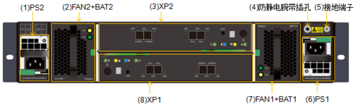
图3-11 SSU2225B 后正视图
