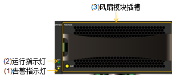
图3-4 SP 正视图
