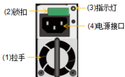
图3-26 DSU2624 电源模块正视图
