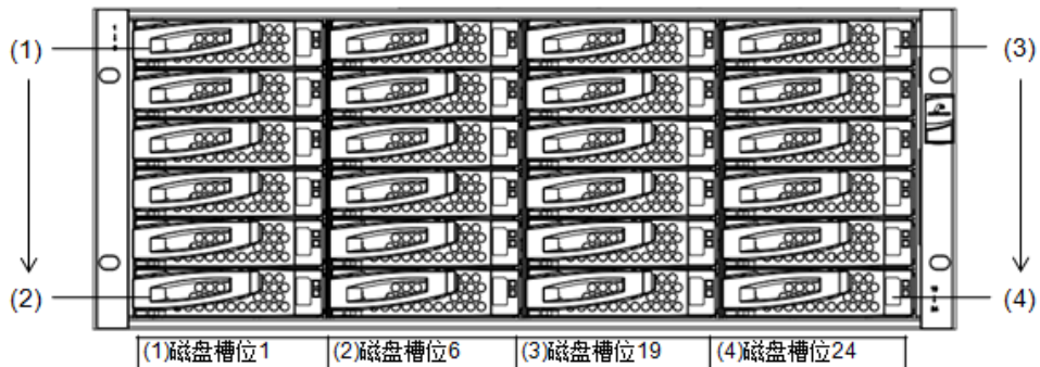
图6-20 DSU2624 磁盘槽位编号示意图
