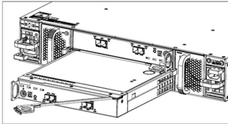
图6-7 安装/拆卸 XP 示意图
