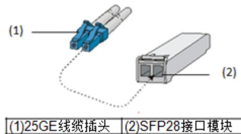
图4-45 25GE 线缆和接口示意图
