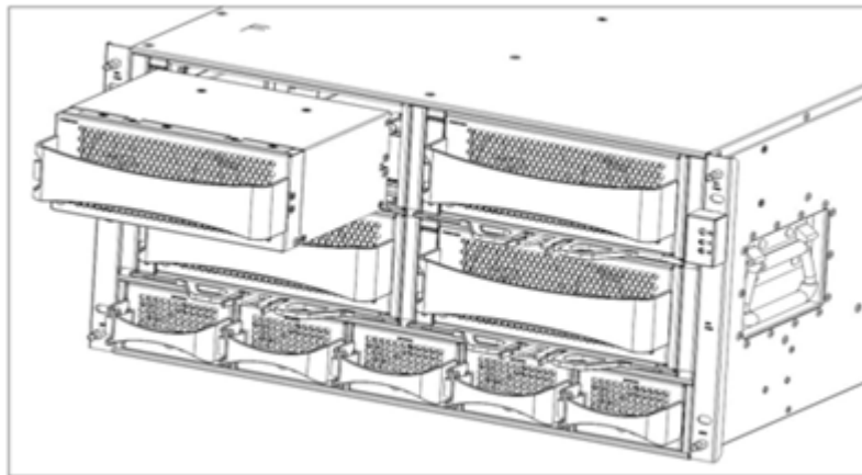
图6-3 安装/拆卸 SPU 风扇模块示意图（一）
