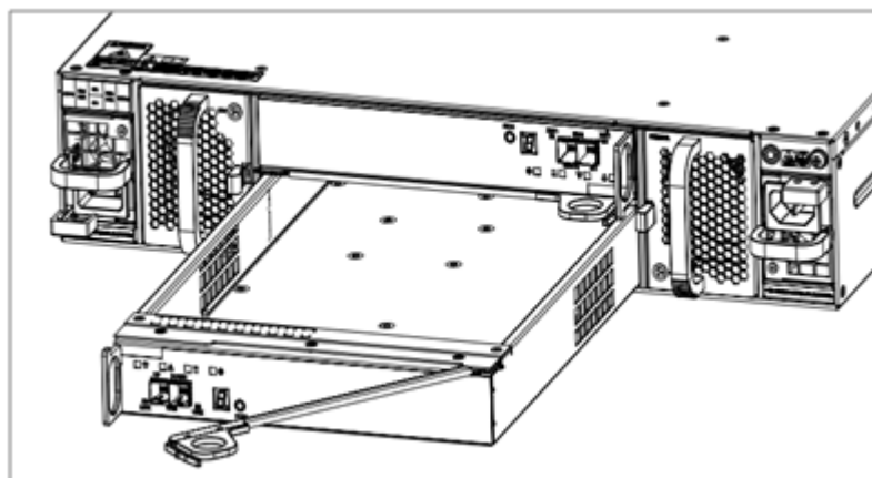
图6-10 安装/拆卸 DSU2625 EP 示意图
