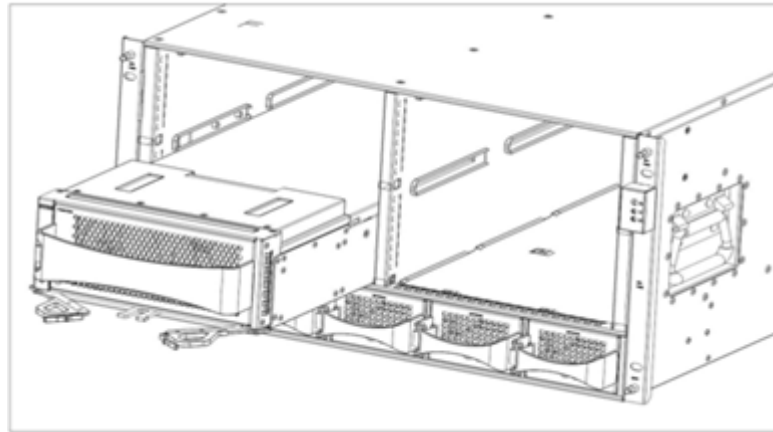
图6-2 安装/拆卸 SP 示意图
