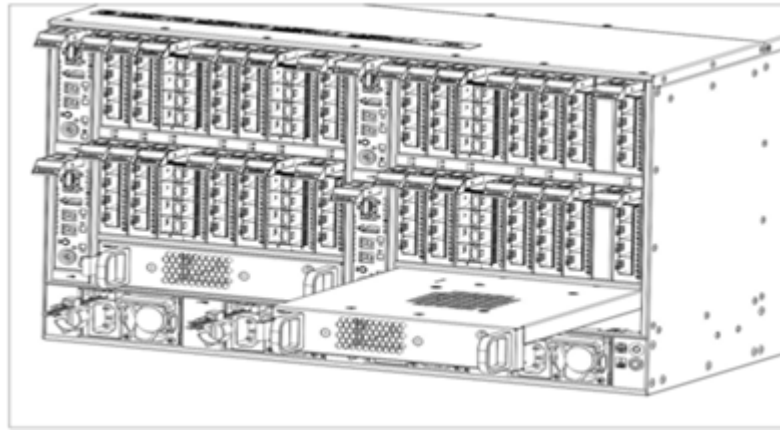
图6-4 安装/拆卸 SPU 风扇模块示意图（二）
