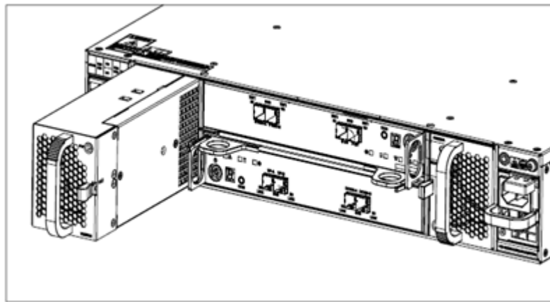
图6-9 安装/拆卸 SSU2225 风扇模块示意图
