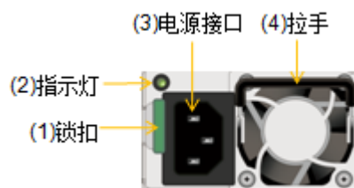
图3-9 SPU 电源模块正视图
