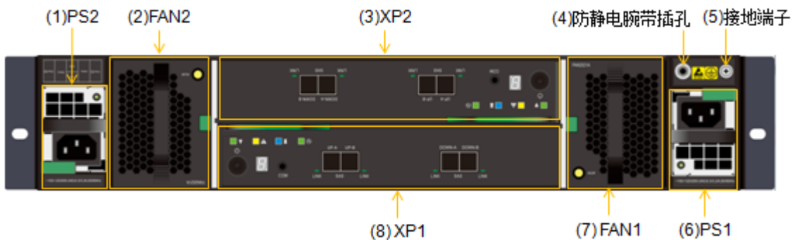
图3-12 SSU2225 后正视图
