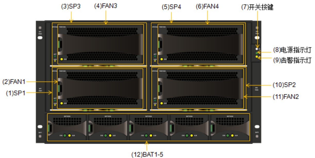
图3-2 SPU 前正视图（不带面板）
