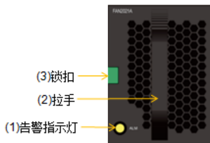
图3-20 DSU2625 风扇模块正视图
