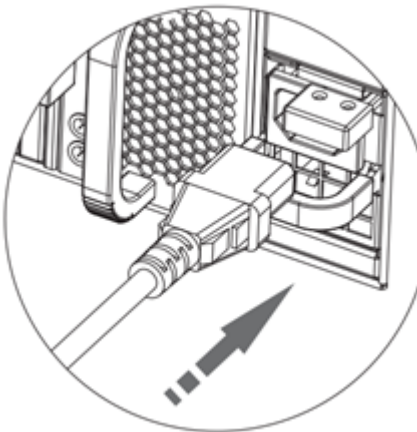
图4-34 安装电源线示意图（三）
