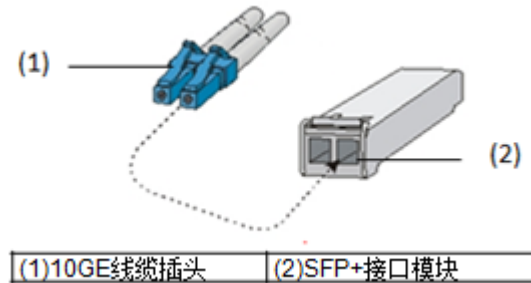
图4-44 10GE 线缆和接口示意图
