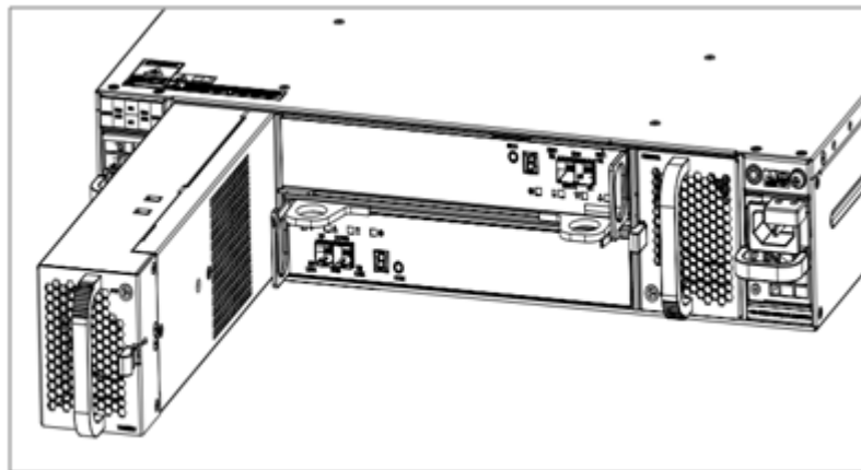
图6-12 安装/拆卸 DSU2625 风扇模块示意图
