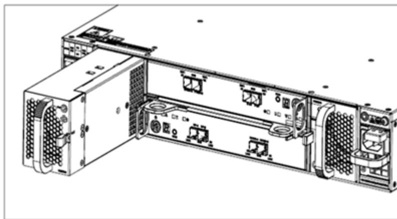
图6-8 安装/拆卸 SSU2225B 风扇模块+电池模块示意图
