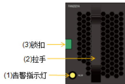
图3-15 SSU2225 风扇模块正视图
