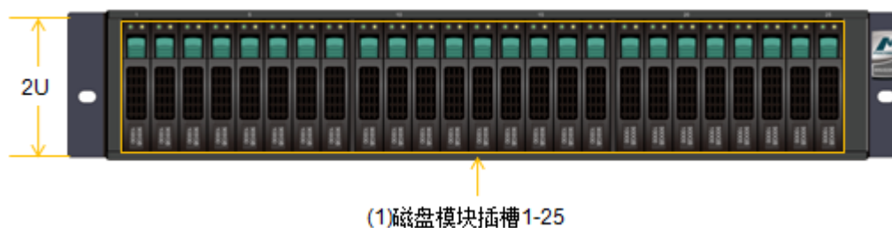
图3-10 SSU 前正视图
