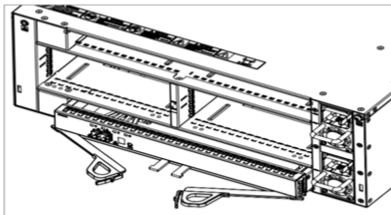
图6-11 安装/拆卸 DSU2624 EP 示意图
