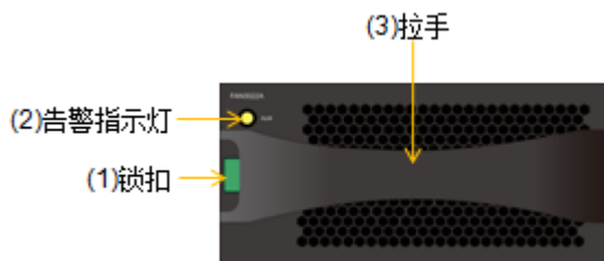
图3-25 DSU2624 风扇模块正视图
