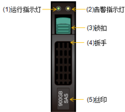
图3-27 2.5 英寸磁盘模块前面板
