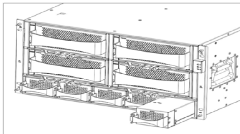
图4-15 安装 SPU 电池模块示意图
