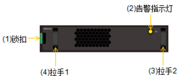
图3-7 SPU 风扇模块正视图（二）
